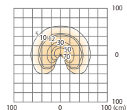
床面照度分布図 ※灯具下向き使用時
