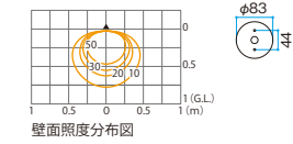
壁面照度分布図
