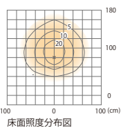
床面照度分布図
