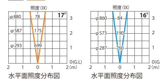
水平面照度分布図
