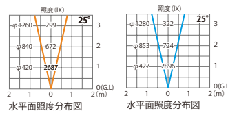
水平面照度分布図
