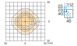
床面照度分布図
