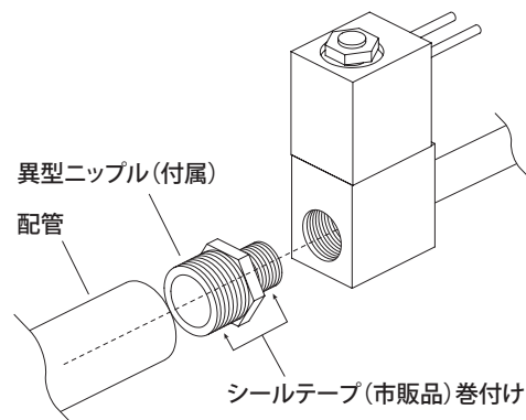
水の入口側
